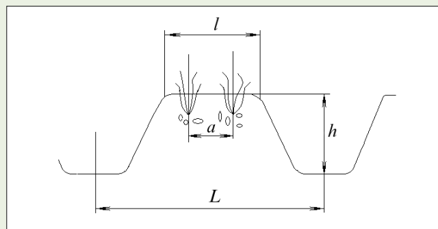
Рис. 1. Форма гряды: a – расстояние между клубнями; L – ширина междурядий; l – ширина вершины гряды; h – высота гряды
