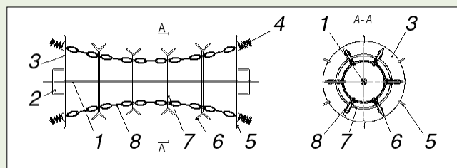
Рис. 2. Схема модернизированной ротационной бороны для обработки гряд:
