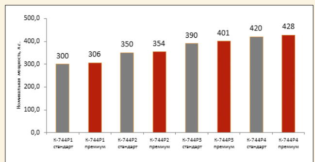
Рисунок. Модульный ряд сельскохозяйственных тракторов «Кировец»
