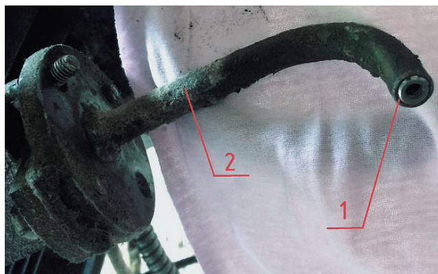
Рис. 3. Форсунка с установленным жиклером: 1 – жиклер; 2 – трубка форсунки
