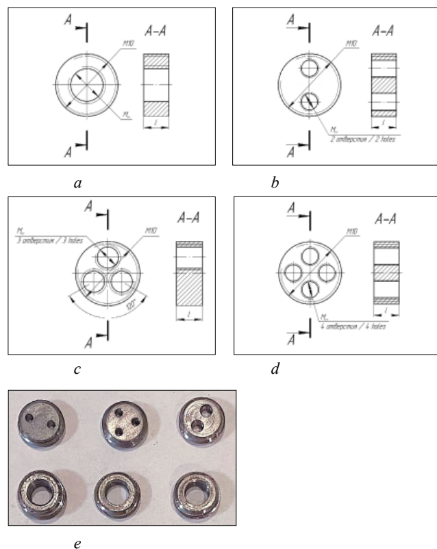
Рис. 2. Схемы жиклеров с разным количеством отверстий: а – с одним; б – с двумя; в – с тремя; д – с четырьмя; е – общий вид работоспособных жиклеров
