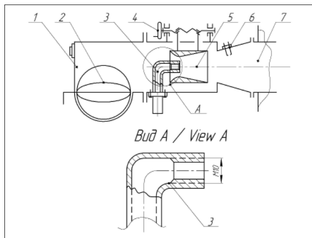
Рис. 1. Схема горелки топочного агрегата ТБМ-1,7: 1 – вентилятор; 2 – заслонка; 3 – трубка форсунки; 4 – маховичок регулировки положения диффузора; 5 – диффузор; 6 – запальная свеча; 7 – топочный агрегат
