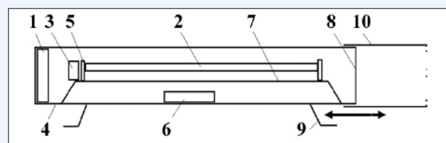
Рис. 1. Устройство АРУФ
